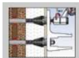
Faza 10: strângeți obiectul de fixat
