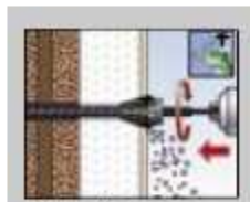
Faza 3: instalați MTH THERMAX cu un burghiu prevăzut cu o inserție hexagonală
