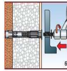
Faza 6: fixați pe capul diblului o eventuală bridă cu șuruburi
