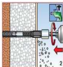
Faza 2: creați un locaș în tencuială și în izolație utilizând MTH THERMAX JUNIOR fără dibluri
