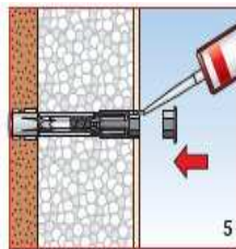
Faza 5: sigilați conturul capului diblului cu un silicon adecvat
