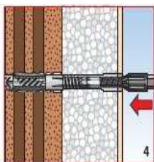
Faza 4: Introduceți diblul astfel încât capul diblului să fie la același nivel cu tencuiala externă
