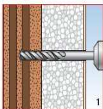
Faza 1: executați o gaură
